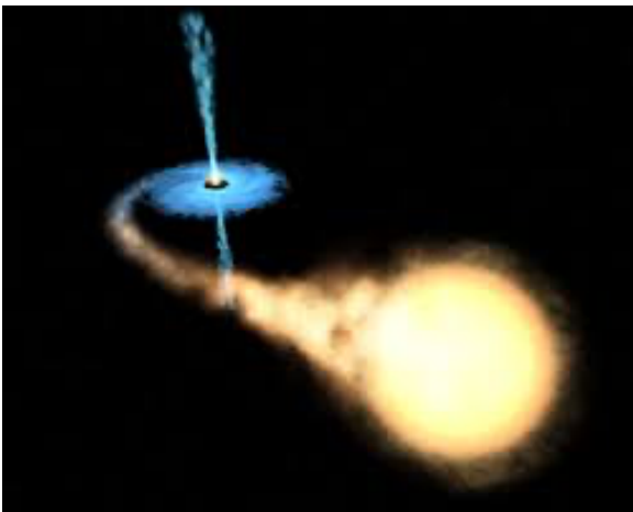
ブラックホール X 線連星の想像図
